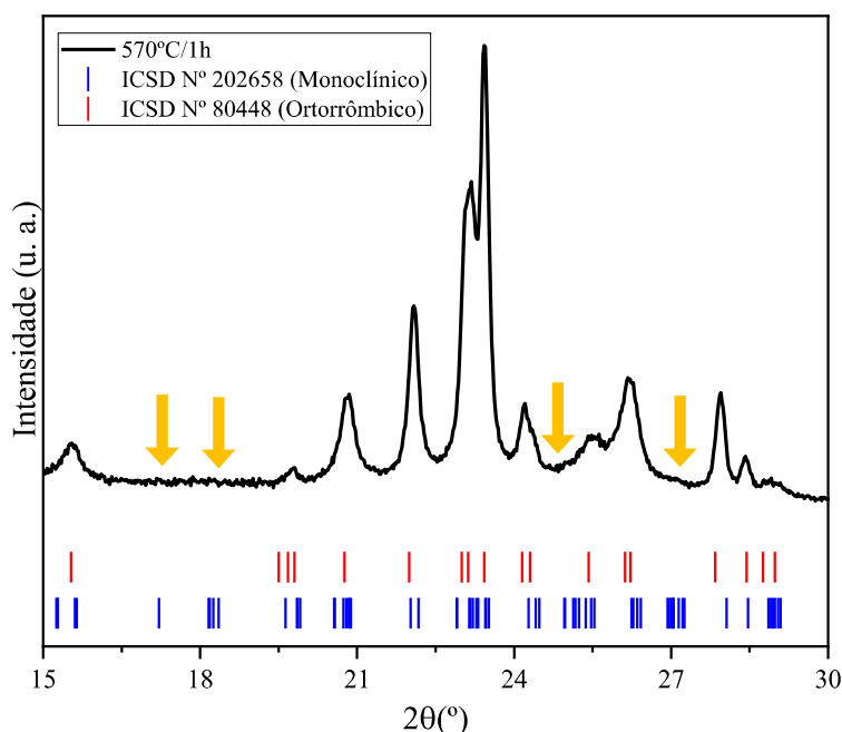
Figura 11: Difratoograma ampliado entre 15 e 30° do precipitado tratado termicamente a 570 °C/1h indexado à fase \alpha e \beta do \text{Al}_2(\text{MoO}_4)_3 .
