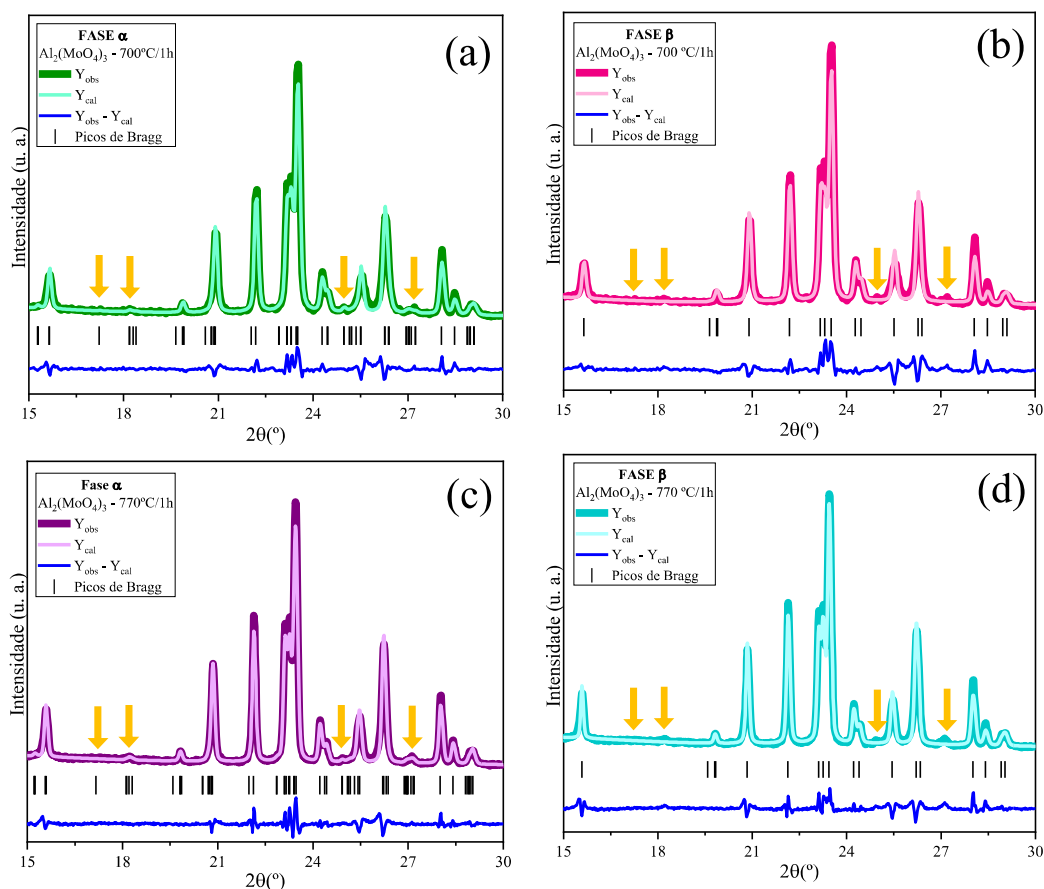
Figura 16: Ampliação do refinamento pelo Método de Rietveld do \text{Al}_2(\text{MoO}_4)_3 tratado termicamente a 700 °C/1h para fase (a) \alpha e (b) \beta e a 770 °C/1h para fase (c) \alpha e (d) \beta entre 15 e 30°.
