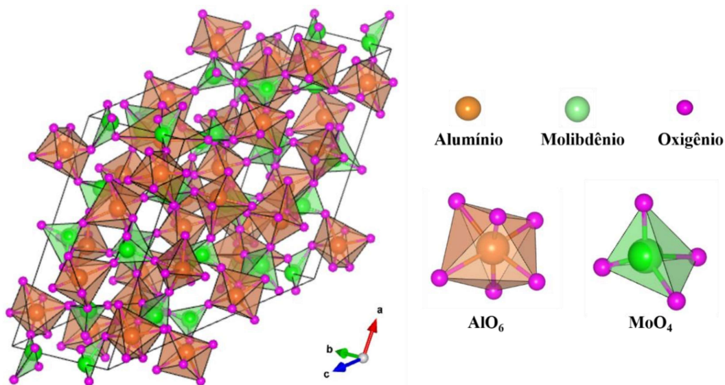
Figura 17: Célula unitária do \text{Al}_2(\text{MoO}_4)_3 tratado termicamente a 700 °C/1h.
