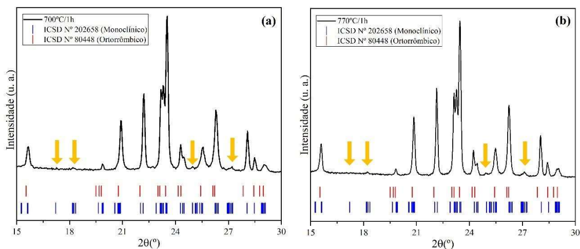
Figura 12: Difratoogramas ampliados entre 15 e 30° do precipitado tratado termicamente a (a) 700 °C/1h e (b) 770 °C/1h indexados à fase \alpha e \beta do \text{Al}_2(\text{MoO}_4)_3 .
