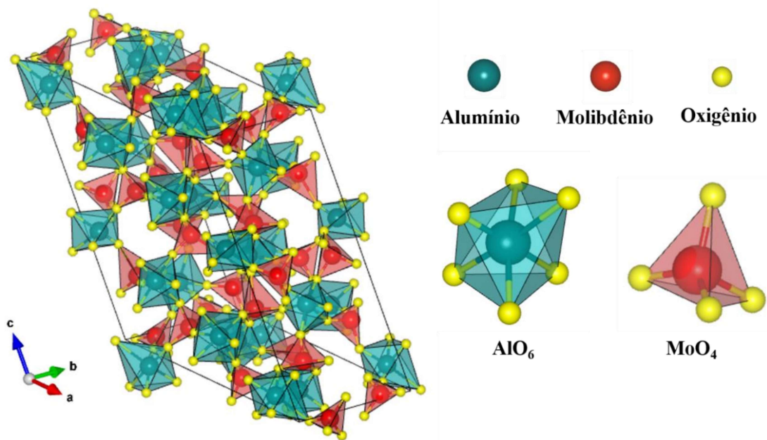
Figura 18: Célula unitária do \text{Al}_2(\text{MoO}_4)_3 tratado termicamente a 770 °C/1h.
